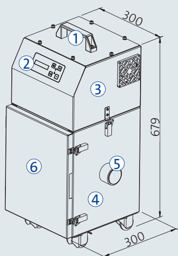
Dessin sans dépoussiérage automatique
